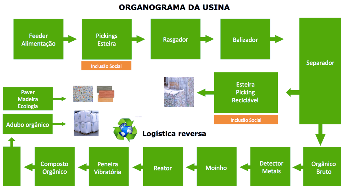
Figura 07 – Organograma da usina de triagem e tratamento de resíduos. Fonte: Sinertec
